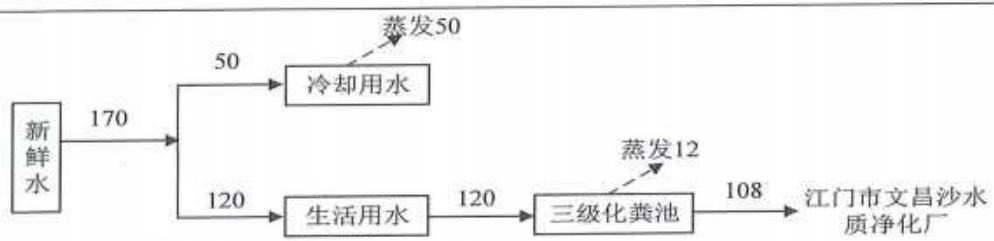
图 1. 水平衡图
