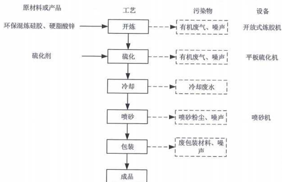
图 2. 密封圈杂件生产工艺流程图
